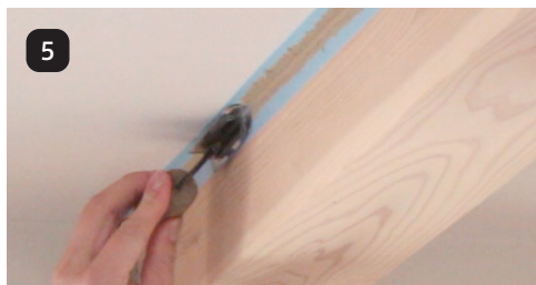
入隅用のコテで入れた珪藻土を押さえます ※隙間に珪藻土が入り込むよう、しっかり押さえて下さい
